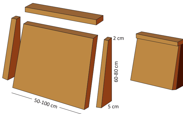
Einfaches Fledermaus- brett als Quartier
